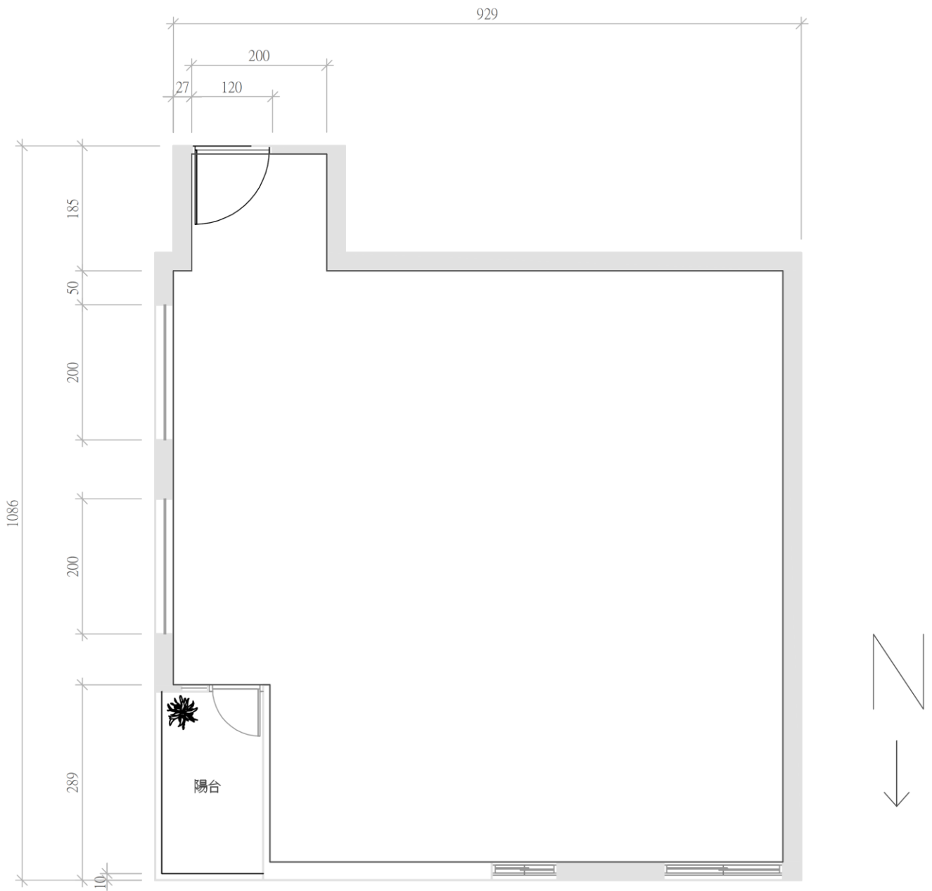
平面圖
